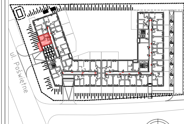
PARTER SCHEMAT - LOKALIZACJA POMIESZCZENIA
